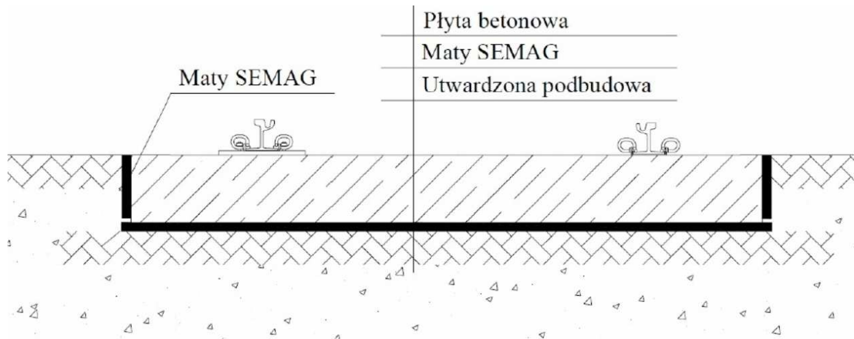
Rysunek Z-2 - Przekrój poprzeczny stosowania maty WM SEMAG w torowiskach o konstrukcji bezpodsypkowej
